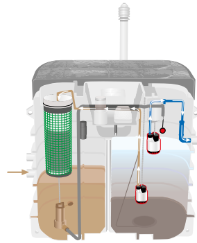
4. Puhdistetun veden poistaminen ja ylijäämälietteen käsittely
