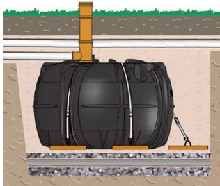
Matalan Uponor-umpisäiliön voit sijoittaa hankalaankin maastoon. Uponor-ankkurointijärjestelmä pitää säiliön tukevasti paikallaan. Kaivanto kannattaa salaajittaa.
