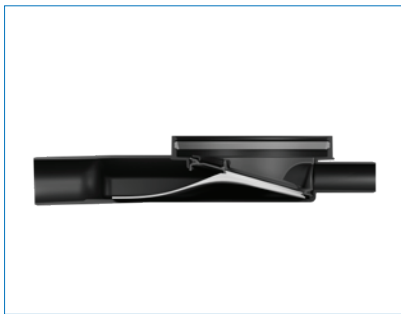
1 Kaivo perustilassa, kalvovesilukko on sulkeutunut.
