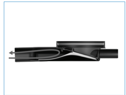
3 Veden tulon loputtua kalvovesilukko sulkeutuu tiiviisti, estäen viemärikaasujen pääsyn huonetilaan.
