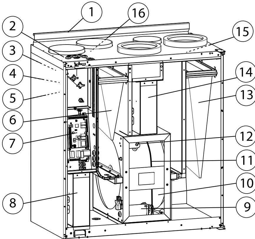
Kuva 11 Sisäiset komponentit
