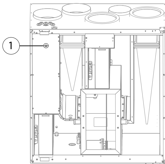
Kuva 12 Ylikuumentumisanturin palautuspainike
