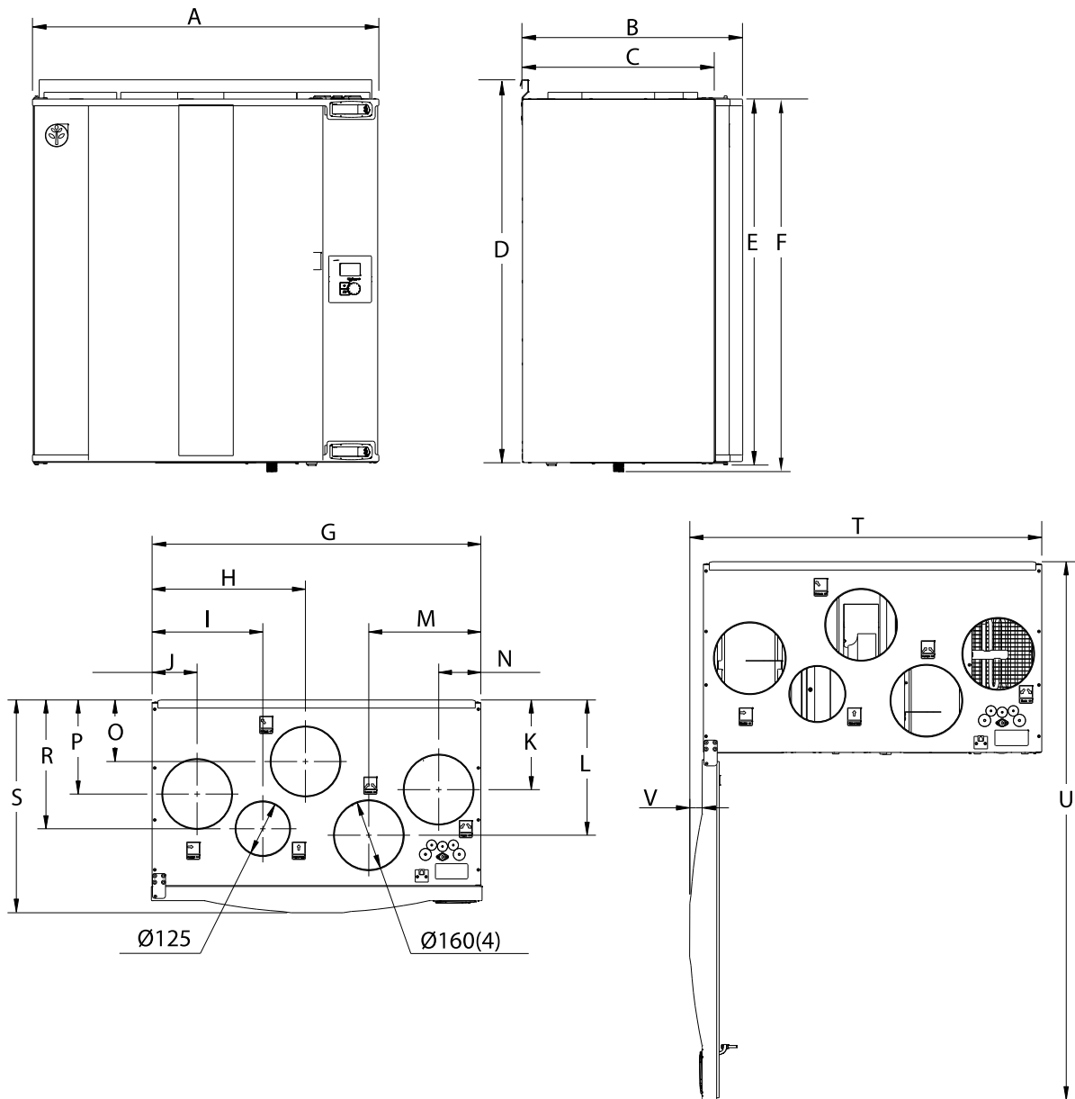
Kuva 2 Mitat ja paino, R-malli
