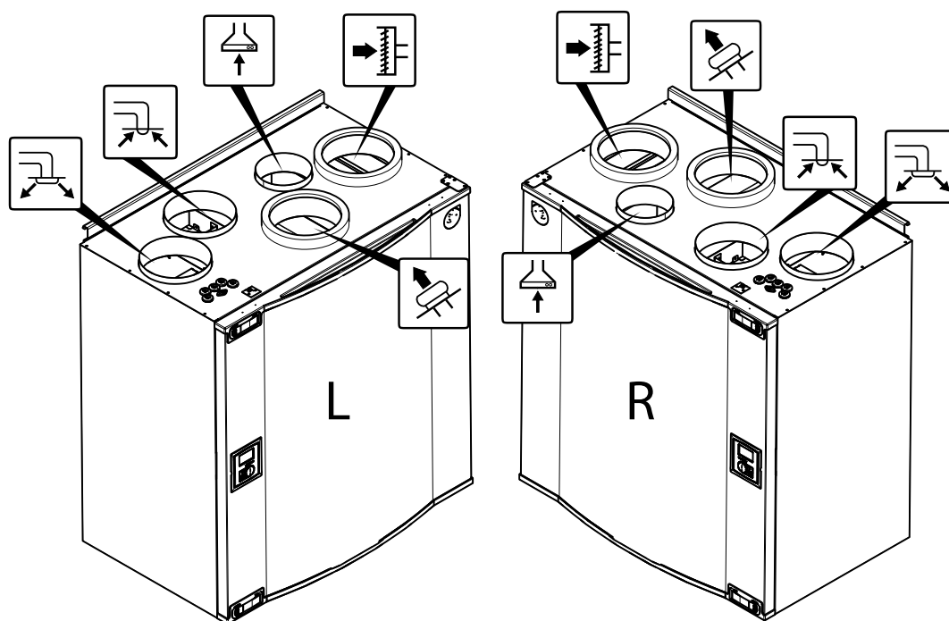
Kuva 3 Kanavaliitännät
