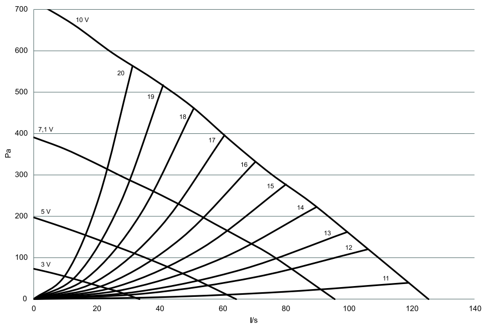
Kuva 6 Tuloilman järjestelmäkäyrät, G3 -tyypin suodatin
