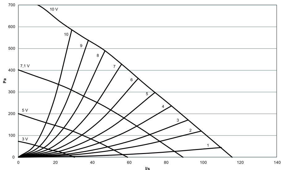
Kuva 7 Poistoilman järjestelmäkäyrät, G3 -tyypin suodatin
