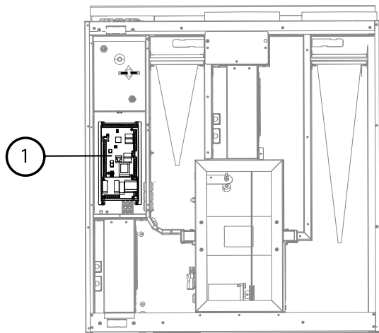
Kuva 8 Piirikortin sijainti
