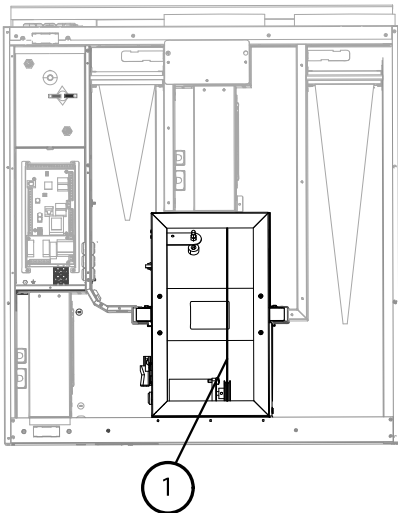
Kuva 13 Roottorin käyttöhihna
