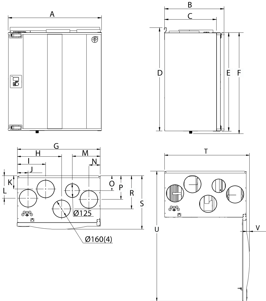
Kuva 1 Mitat ja paino, L-malli
